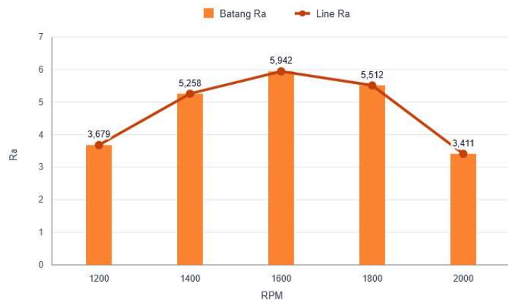
Grafik 4. Kecepatan Spindel vs Ra
