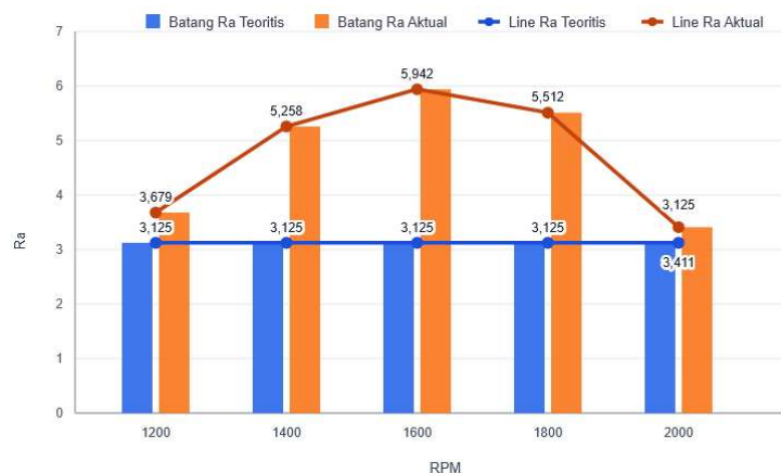
Grafik 1. Perbandingan Ra Teoritis dan Ra Aktual
