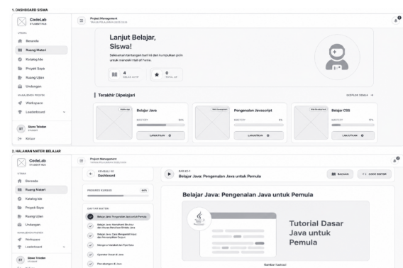
Gambar 9. Wireframe Materi Siswa
